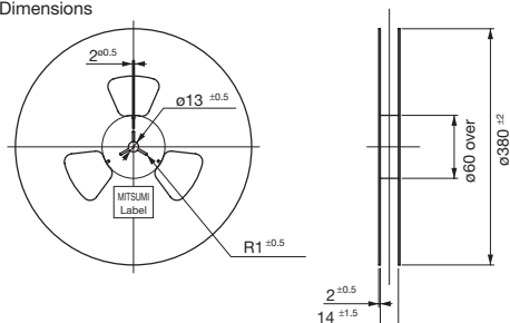
Reel Dimensions
