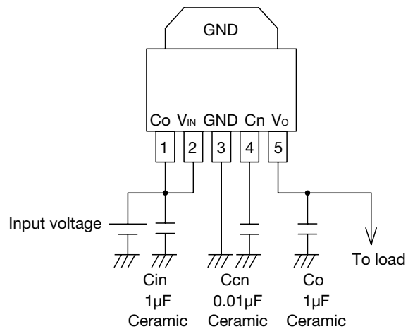
■ TO-252-5A
